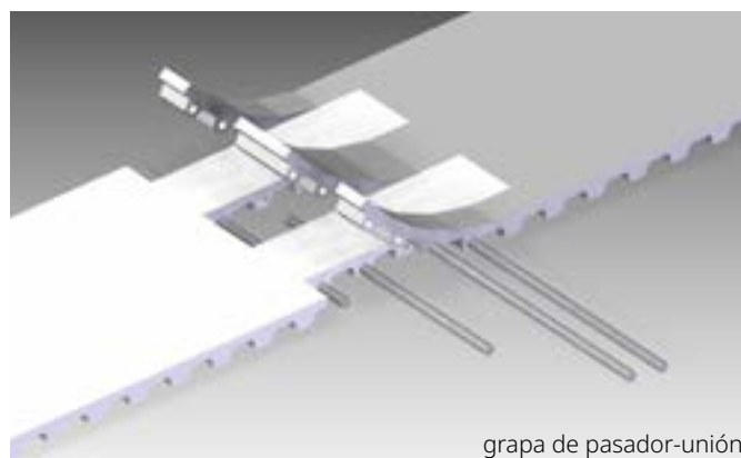
agarre mecánico de los arastradores, dientes metálicos
