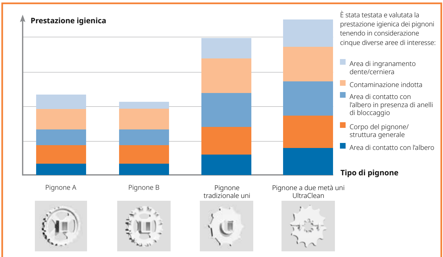
E' stata definita una apposita procedura per riprodurre le condizioni di utilizzo, pulizia e valutazione di pignoni con differenti disegni.
